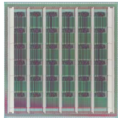
PCA 回路構成を自己変更できるLSI
